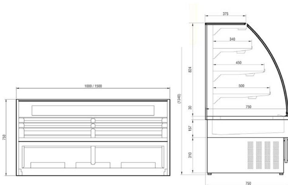
Technický výkres
